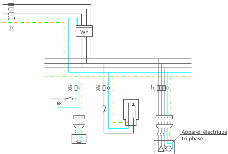
Nouvelle installation en TN-S
