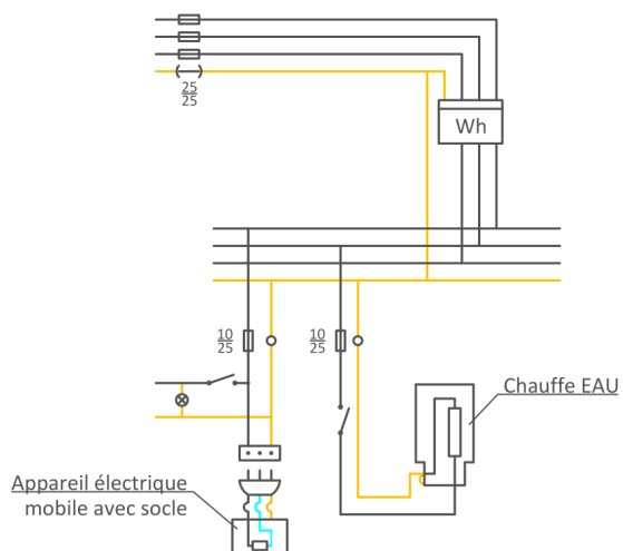
Ancienne installation en schéma III
